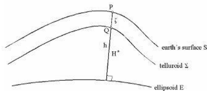
El teluroide. La altura normal= H^* y la altura anómala \zeta
